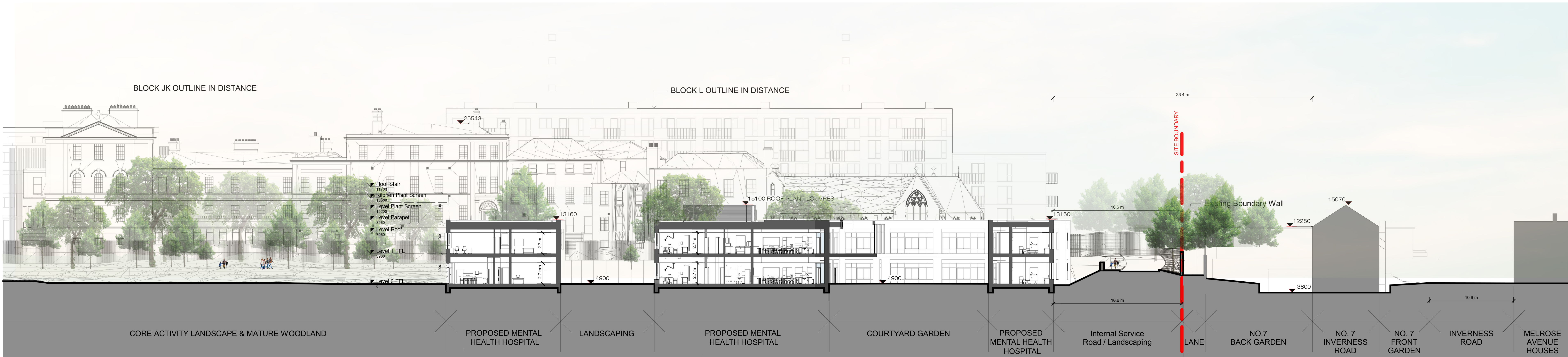
4 Site Section 4-4 SCALE: 1 : 200
