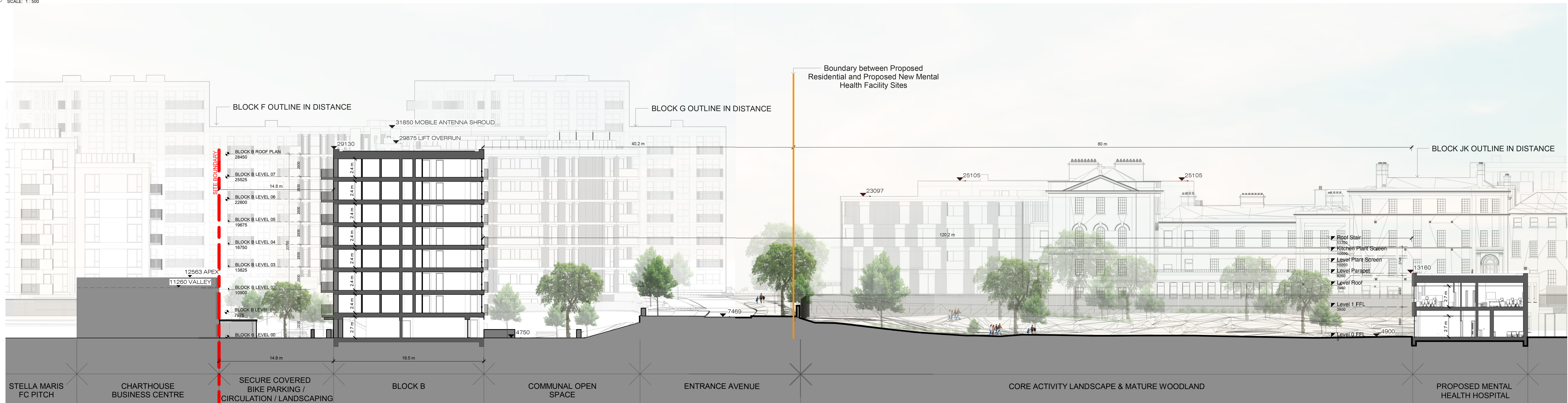
3 Site Section 3-3 SCALE: 1 : 200
